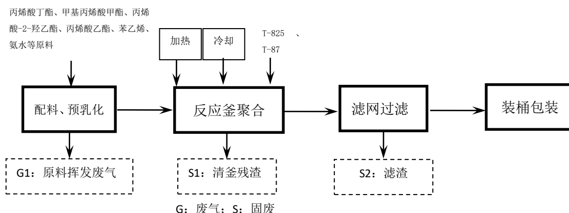
图 4-4 无溶剂粘合剂生产工艺流程图
